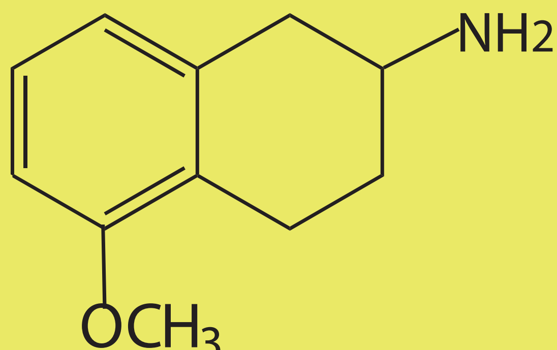
5-Methoxy 2-AminotetralinHCL
