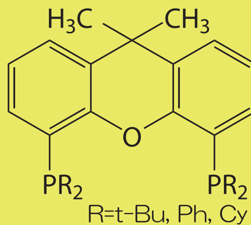
XANTHPHOS, 99%
