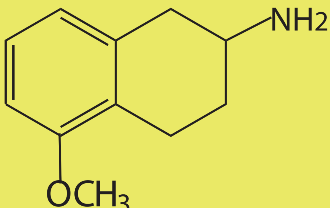
5-Methoxy 2-AminotetralinHCL
